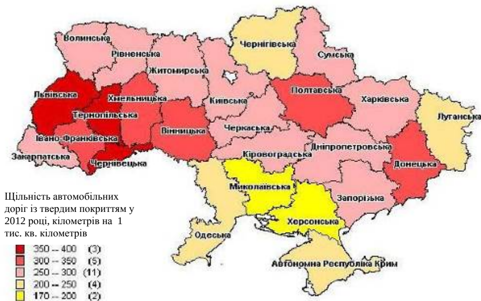
Рис. 32. Щільність автомобільних доріг із твердим покриттям
